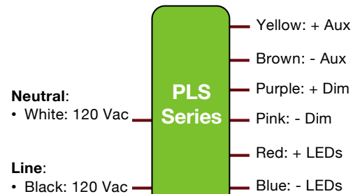
Wiring Diagrams
